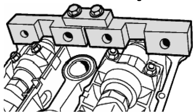
Nockenwelle-Arretierung
