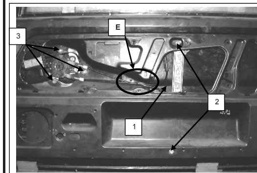
Porta lato destro, Portière avant droite, Right front door, Puerta lado derecho, Vorne rechte Tür, Porta frente dirieta, Sag on kapı, πόρτα εμπρόσθια δεξιά
