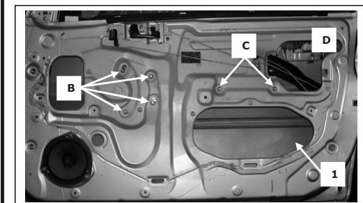
Porta lato destro, Portière avant droite, Right front door, Puerta lado derecho, Vorne rechte Tür, Porta frente diarieta, Sag on kapi, πόρτα εμπρόσθια δεξιά
