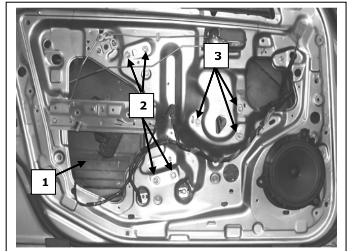
Porta lato destro, Portière avant droite, Right front door, Puerta lado derecho, Vorne rechte Tür, Porta frente dirieta, Sag on kapi, πόρτα εμπρόςα δεξιά
