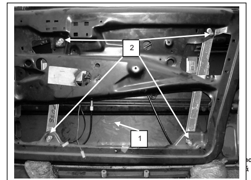
Alzacristallo originale - oem window regulator - lève-vitre original - Fensterheber von oem - elevalunas original - levandador de vidro original - oriijnal cam acacagi - Γρύλος γνήσιος Nostro alzacristallo - our window regulator - notre lève-vitre - unser Fensterheber - nuestro elevalunas - nosso levantador de vidro - bizim cam acacagi - Γρύλος δικός μας
