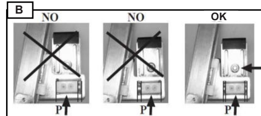
Porta lato destro, Portière avant droite, Right front door, Puerta lado derecho, Vorne rechte Tür, Porta frente dirieta, Sag on kapi, πόρτα εμπρόςθια δεξιά
