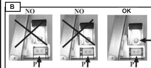
Porta lato sinistro, Portière avant gauche, Left front door, Puerta lado izquierdo, Vorne links Tür, Porta frente esquerda, Sol on kapi, πόρτα εμπρόςθια αριστερή
