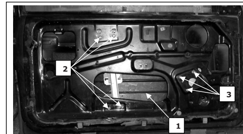
Porta lato sinistro, Portière arrière gauche, Left rear door, Puerta lado izquierdo, Hinten links Tür, Porta traseira esquerda, Sol arka kapi, πόρτα οπίσθια αριστερή
