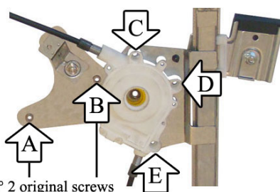
A POWER WINDOW LEFT ALZACRISTALLI ELETTRICO SX
