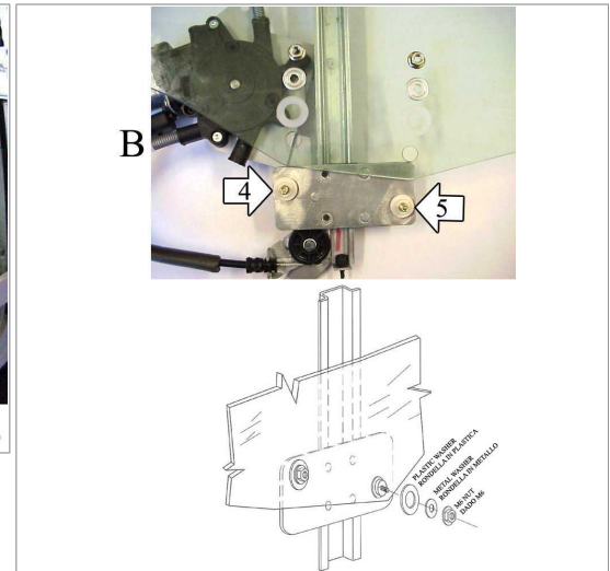
2 Doors - 2 Portes - 2 Türlig - 2 Puertas - 2 Porte right door - portière droite - rechte tür - puerta lado derecho - porta lato destro
