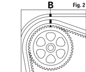
FIGURA 1 Verificar que la marca de puesta a tiempo este en línea con la marca del cárter de la distribución A. FIGURA 2 Verificar la correcta alineación de las marcas de puesta en fase B.
