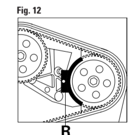
FIGURA 11 Controllare il corretto allineamento delle tacche di fase O. FIGURA 12 Inserire l'apposito attrezzo di bloccaggio della puleggia della pompa di iniezione R.
