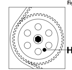
FIGURA 6 Inserire l'apposito attrezzo di bloccaggio della puleggia della pompa di iniezione H.
