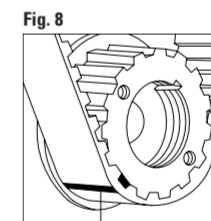
FIGURA 8 Controllare il corretto allineamento delle tacche di fase I. FIGURA 9 Inserire l'apposito attrezzo di bloccaggio dell'albero motore L.
