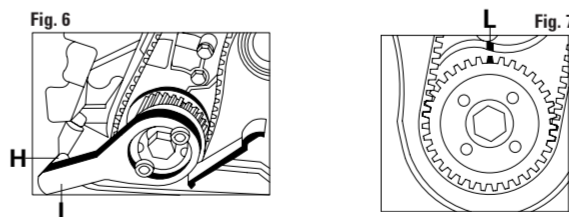
FIGURA 6 Extraer el tornillo del cárter frontal H e insertar la herramienta específica para inmovilizar el cigüeñal I. FIGURA 7 Verificar la correcta alineación de las marcas de puesta en fase L.
