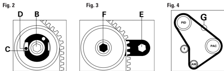
FIGURA 2 Per motori non turbo: allentare il bullone di bloccaggio B e ruotare in senso orario il tendicinghia fino ad allineare la tacca C con la tacca D, quindi, serrare il bullone di bloccaggio B. FIGURA 3 Per motori turbo: allentare i bulloni di bloccaggio E ed F del tendicinghia. FIGURA 4 Per motori turbo: premere sulla parte indicata G fino alla giusta tensione e serrare, quindi, i bulloni di bloccaggio F ed E.
