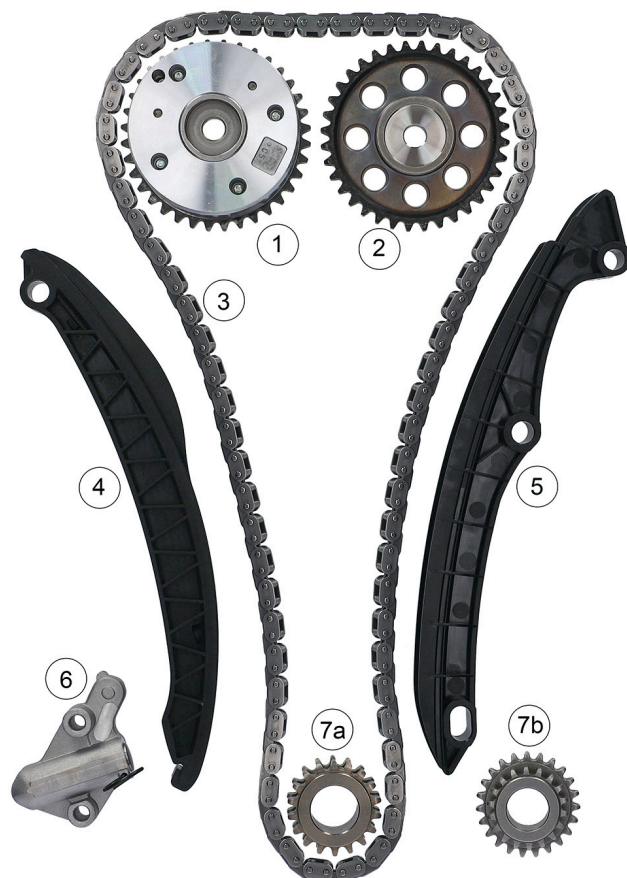
Снимка 1: 559 0154 30/559 0154 31 – Компоненти за комплект ангренажна верига
