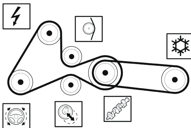
Figuur 2: Hulpaggregaataandrijving vanaf motornummer 0113090 met elastische multiriem
