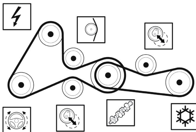
Figuur 1: Hulpaggregaataandrijving tot motornummer 0113089 met spanrol
