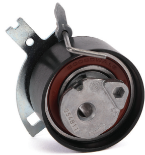
Resim 1: 531 0810 10 gergi rulmanı
