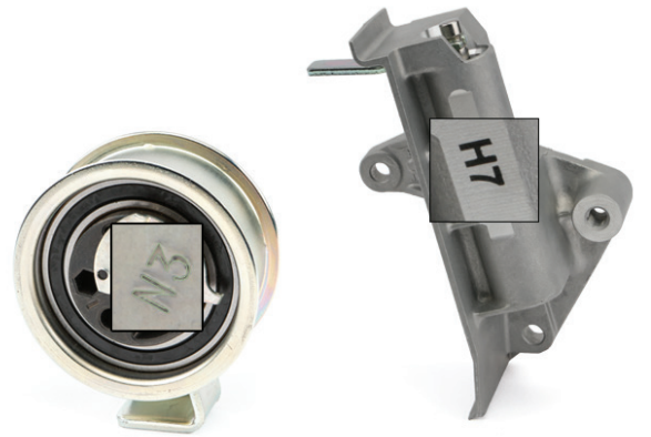
Resim 1: 531 0396 20 gergi rulmanı, 533 0039 10 titreşim damperisi ile birlikte
