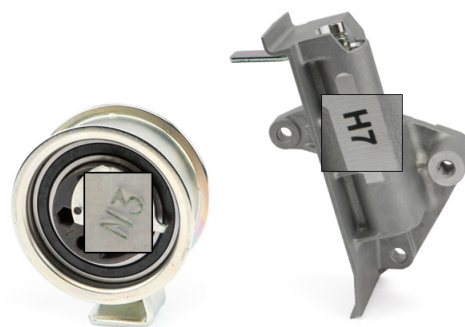
Bild 1: Spännrulle 531 0396 20 med vibrationsdämpare 533 0039 10
