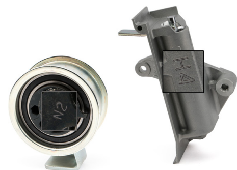
Bild 2: Spännrulle 531 0436 20 med vibrationsdämpare 533 0035 10
