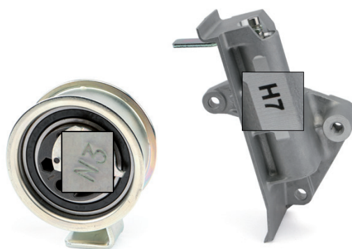
Figura 1: Rullo tenditore 531 0396 20 con smorzatore di vibrazioni 533 0039 10
