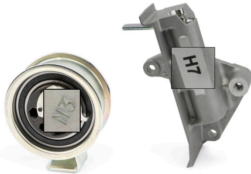
איור 1: גלגלת מותחן מק"ט – 531 0396 20 בעלת משכך רעידות מק"ט – 533 0039 10
