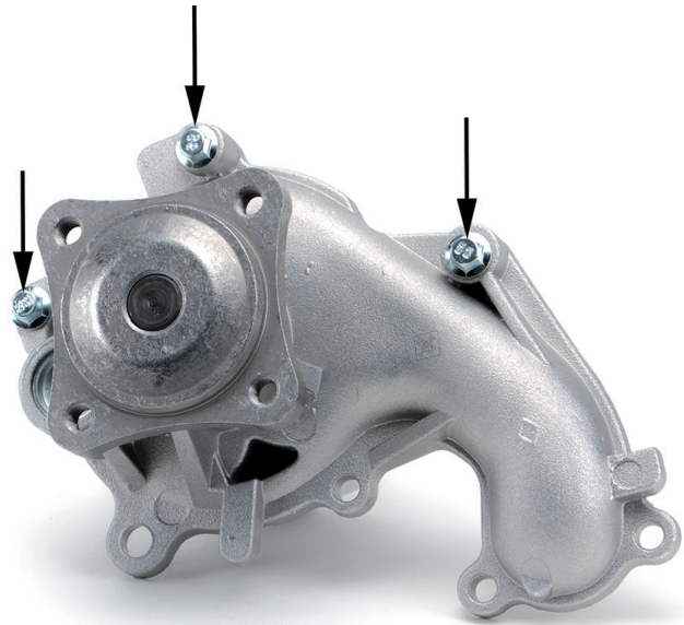
Figura 2: Punti di fissaggio modificati della pompa del liquido di raffreddamento
