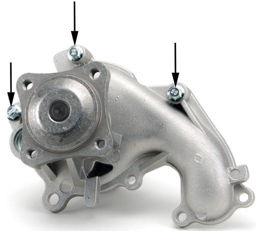
Kuva 2: Jäähdytysnestepumpun modifioidut kiinnityspisteet
