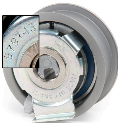
Figura 1: 531 0777 10 – vechea rolă de întindere (979743)
