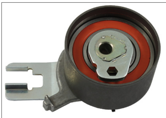
Photo 2: 531 0515 10 – Ancien galet tendeur
