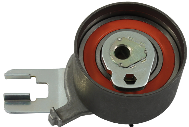
Kuva 2: 531 0515 10 – vanhaa hihnankiristin
