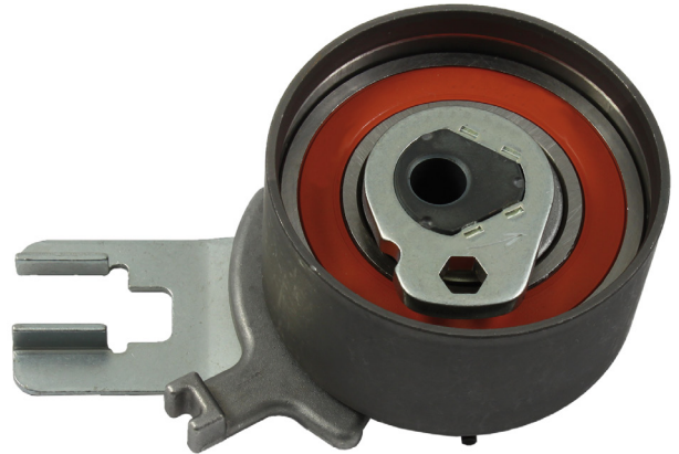
Kuva 1: 531 0859 10 – uusi hihnankiristin
