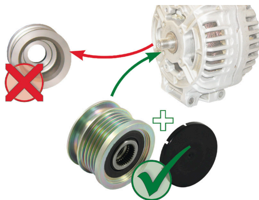
Obrázek 1: Výměna pevné řemenice za alternátorovou volnoběžku
