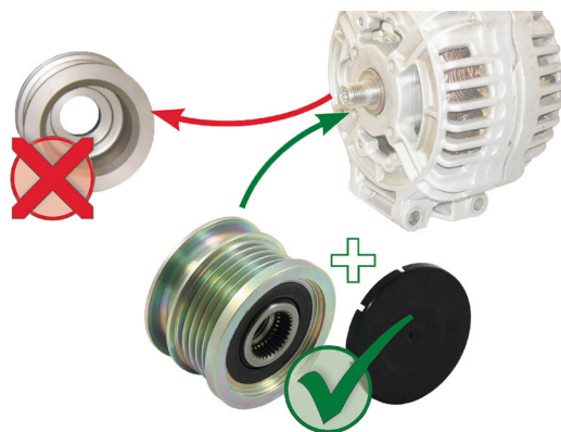
Снимка 1: Промяна от твърда ремъчна ролка към ролка за свободен ход на алтернатор
