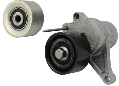
Resim 1: Metal gergi rulmanı ve saptırma kasmağı
