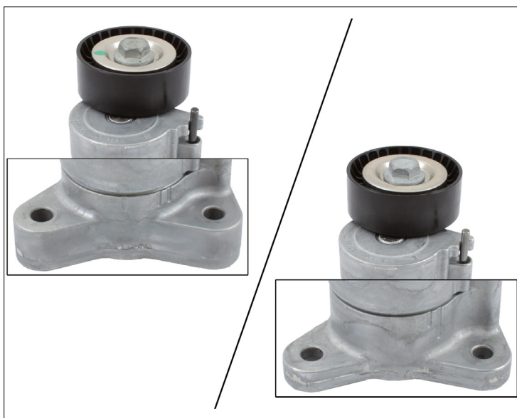
Slika 3: Levo: prejšnja izvedba s širokima pritrditvenima mestoma. Desno: nova izvedba z ozkima pritrditvenima mestoma.
