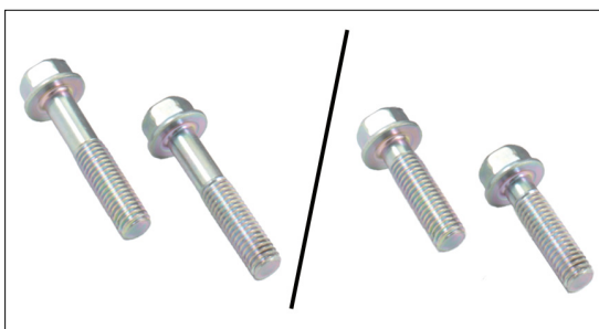
Slika 4: Levo: prejšnja vijaka M8 x 40 mm. Desno: nova vijaka M8 x 30 mm.
