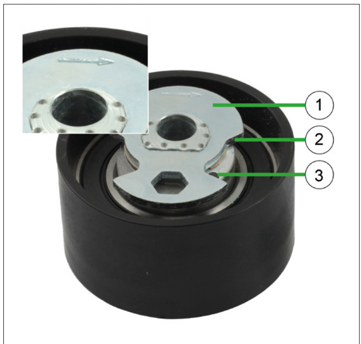
Fig. 1: 531 0504 10 – halfautomatische spanrol
