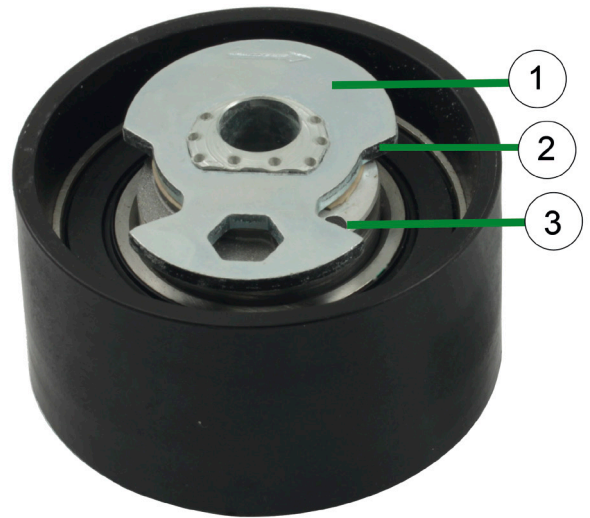
Εικόνα 1: 531 0504 10 – ημι – αυτόματη τροχαλία τάνυσης
