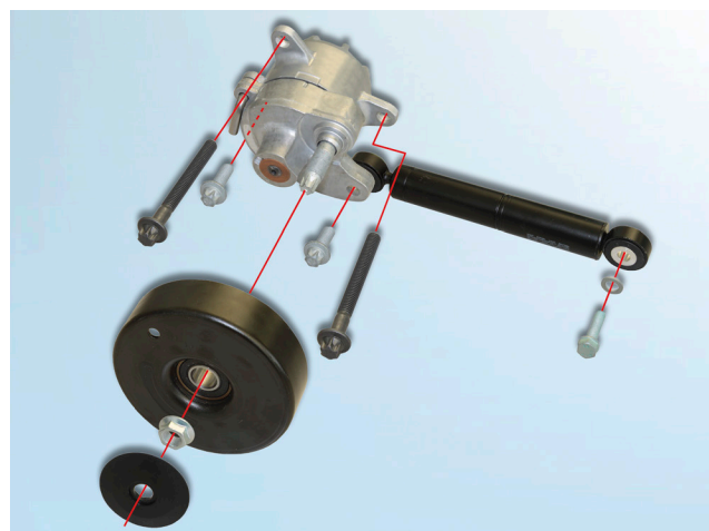
Billede 1: 533 0116 10 – INA reparationssæt til aggregatdrift inkl. fastgøringsskruer
