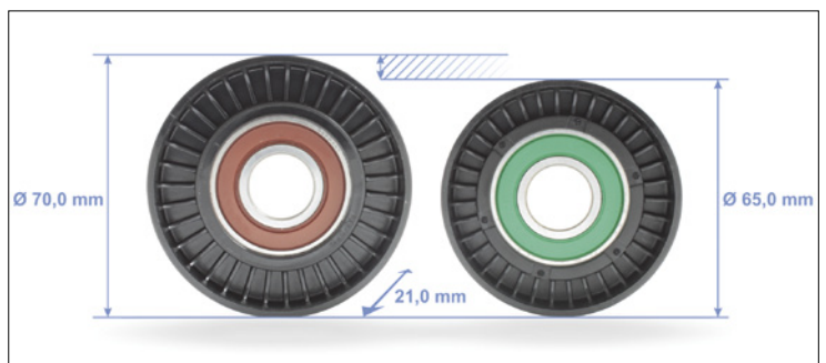
Photo 2 : Poulie de renvoi réf. 532 0404 30 pour véhicules avec moteur essence (à gauche) et poulie de renvoi réf. 532 0406 30 pour véhicules avec moteur diesel (à droite).
