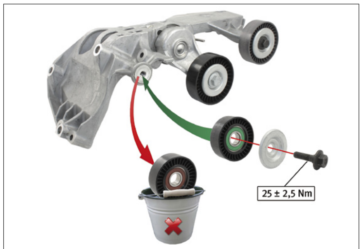
Photo 1 : Bloc tendeur réf. 534 0243 10
