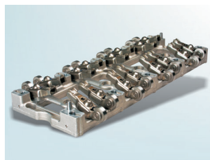
Зображення 1: Блок коромисел 423 0061 10
