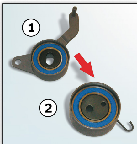
Slika 1: Nadomeščena izvedba napenjalne jermenice 531 0166 20 (1) ter njena naslednica 531 0819 10 (2)
