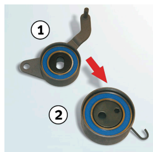
Рисунок 1: Замена натяжного ролика 531 0166 20 (1) на 531 0819 10 (2)
