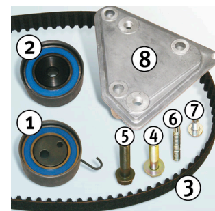
Рисунок 2: Состав упаковки 530 0492 10
