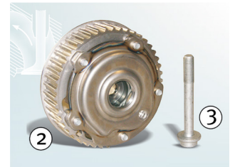
Kuva 2: (2) Pakopuolen hihnapyörä 427 1005 10 ja (3) kiinnitysruuvi (M10x80) 41301*
