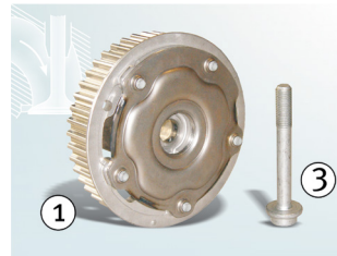
Kuva 1: (1) Imupuolen hihnapyörä 427 1004 10 ja (3) kiinnitysruuvi (M10x80) 41301*
