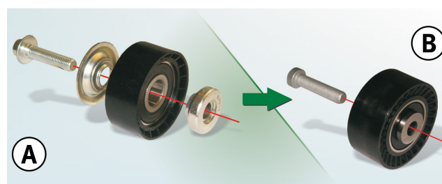
Brytrulle 532 0433 10, tidigare utförande (A) och nytt utförande (B)
