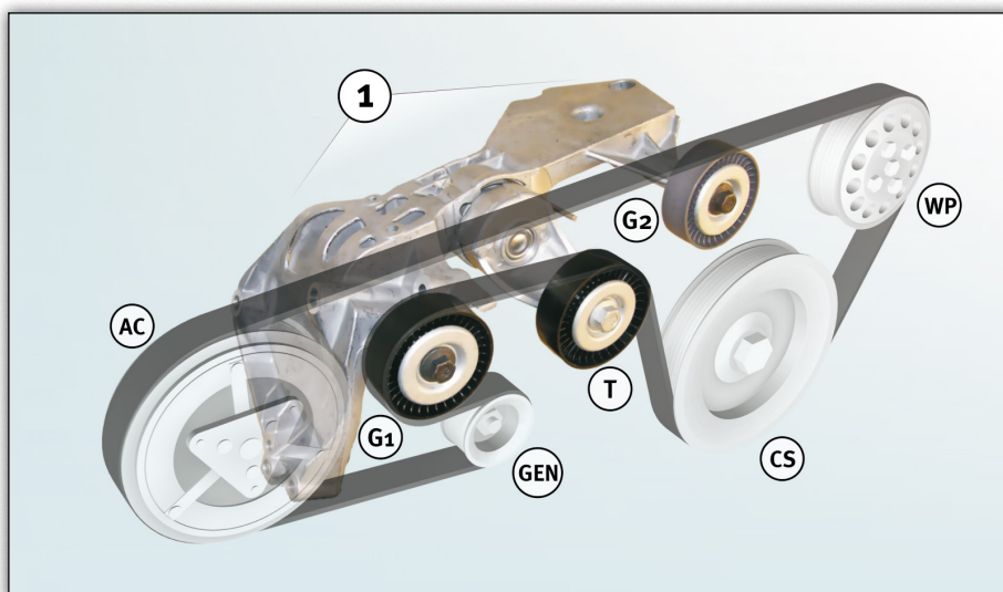
Slika 1: 534 0243 10 - nosilec z napenjalno napravo s pogonom agregatov in pogonska shema
