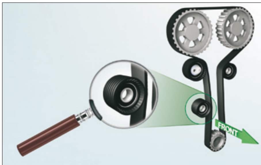
Fig. 1: Riemverloop en rolposities in F4R-motor
