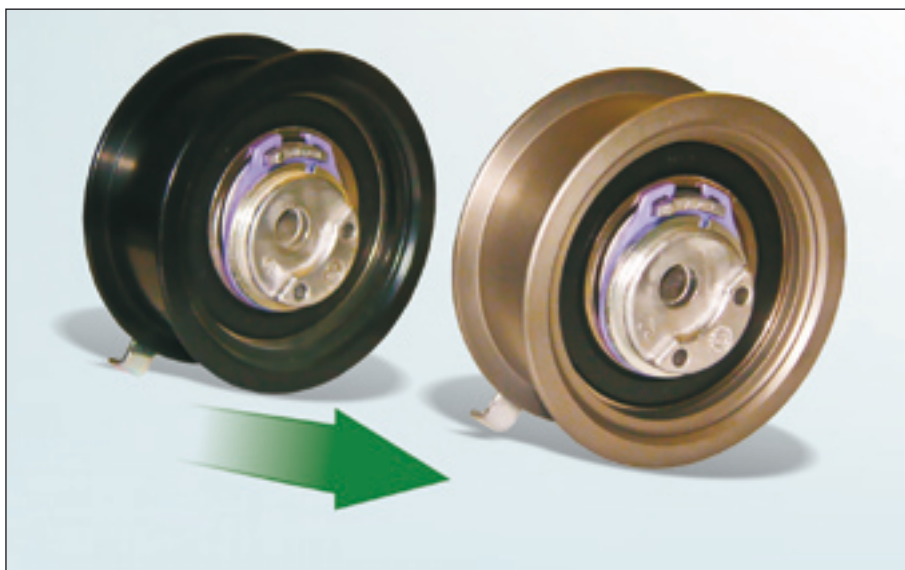
Fig. 1: Verbeterde coating van de loopbaan - hier als voorbeeld getoond op artikelnr. 531 0524 30
