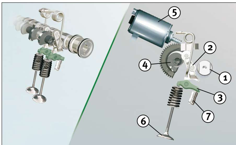
Obrázok 1: Prehľad systému BMW-Valvetronic/detailný pohľad na systémové komponenty
