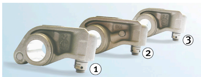
Зображення 1: Огляд трьох різних комплектів коромисел
