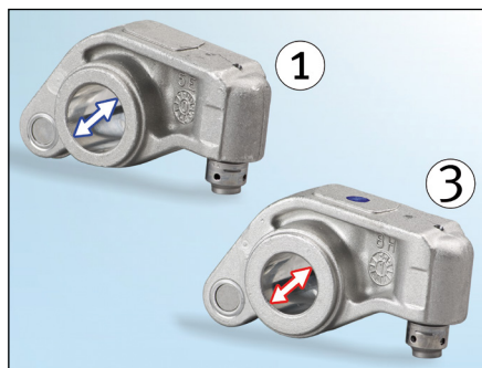
Slika 2: Premer nihajnega vzvoda na sesalni strani (1) je večji
