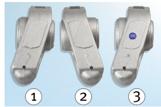
3. ábra: A szelepemelők hajlítása
