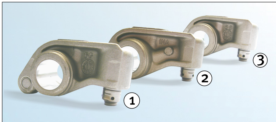
Slika 1: Pregled tri razna KIT-a poluga ventila
