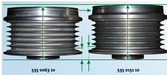
Figura 3: Deosebirea roților libere pentru alternator INA 535 0063 10 (VALEO) și 535 0151 10 (DENSO)
