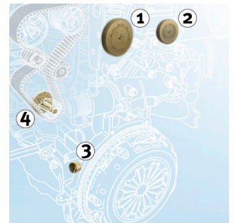
Зображення 2: Монтажне положення
